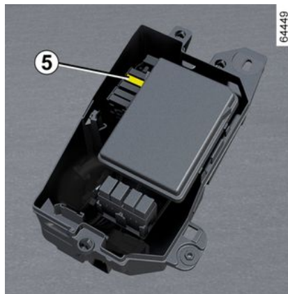
5. Sicherung: Unterbrechung des LPG-Kreislaufs.
